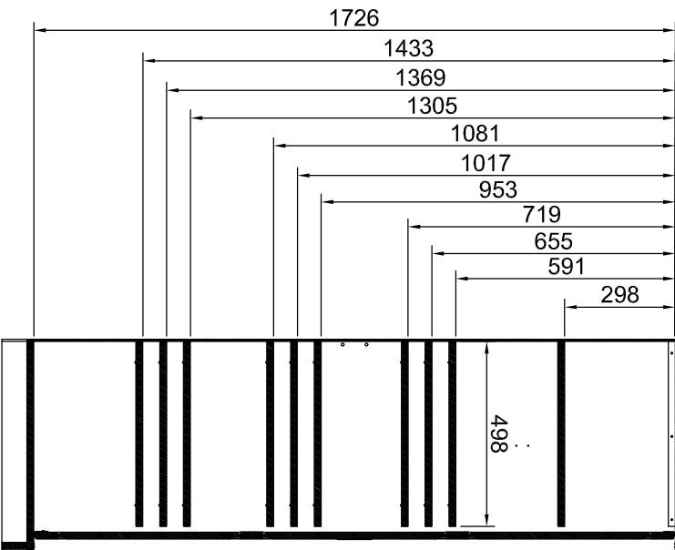
Corte B-B
