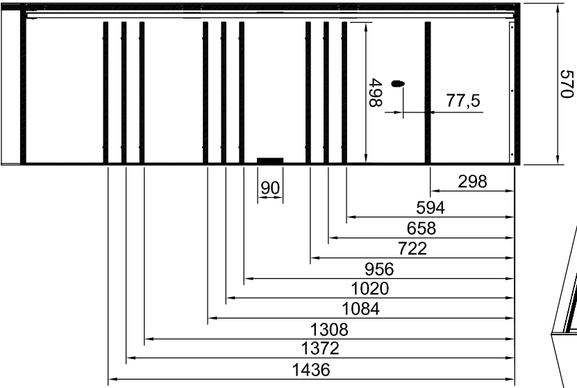
Corte A-A
